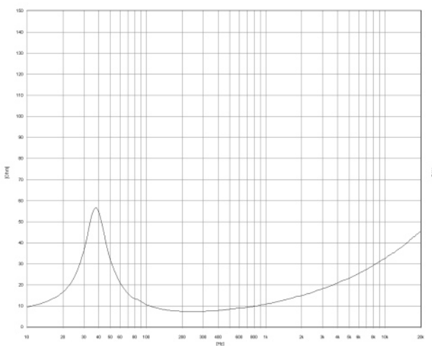
Impedanz Impedance
