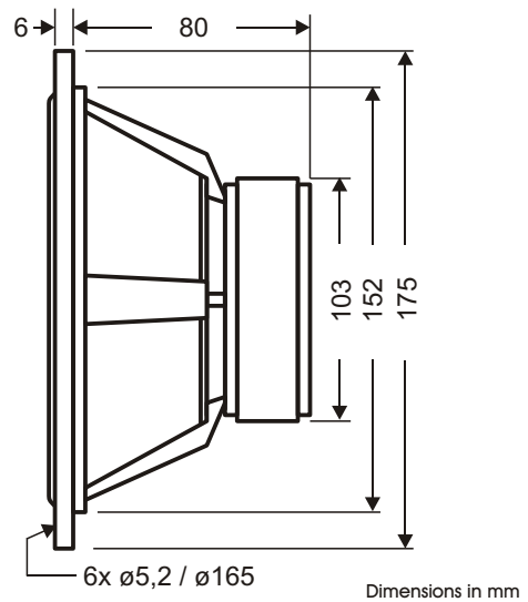
Maße Dimensions
