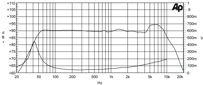
AUDIO PRECISION : W14RC25-04
